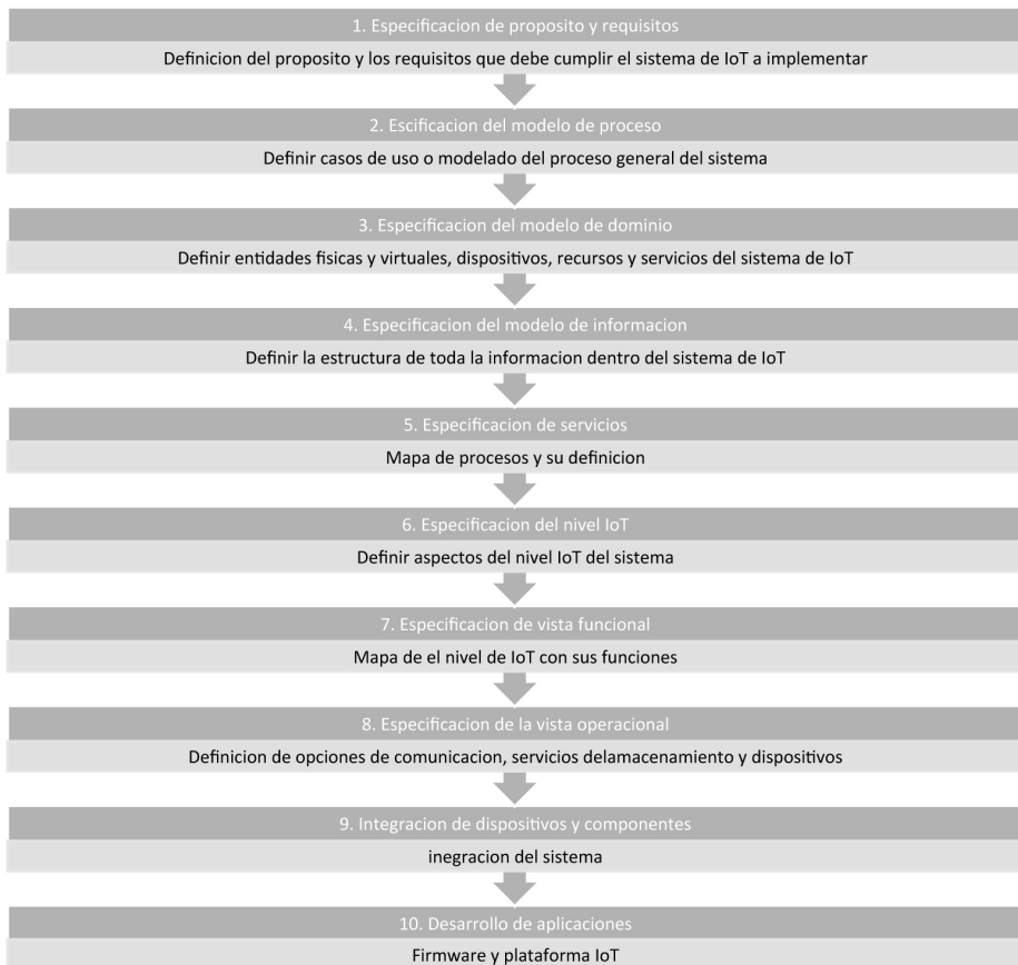
Figura 11. Etapas de la metodología de referencia arquitectural de un sistema IoT (Bahga, 2014)
