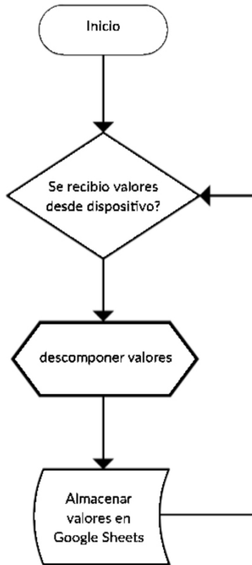
Figura 18. Flujograma general del script para la plataforma IoT del sistema desarrollado. Fuente: diseño propio.
