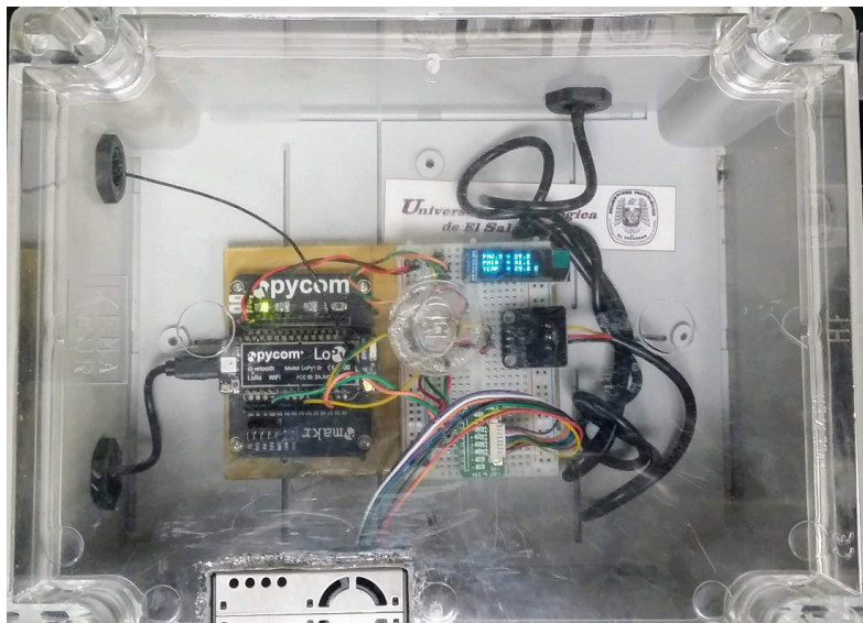
Figura 22. Vista al interior de la carcasa del nodo Iot del sistema diseñado. Fuente: diseño propio.
