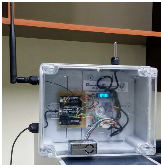
Figura 23. Vista externa completa del nodo IoT del sistema diseñado. Fuente: diseño propio.
