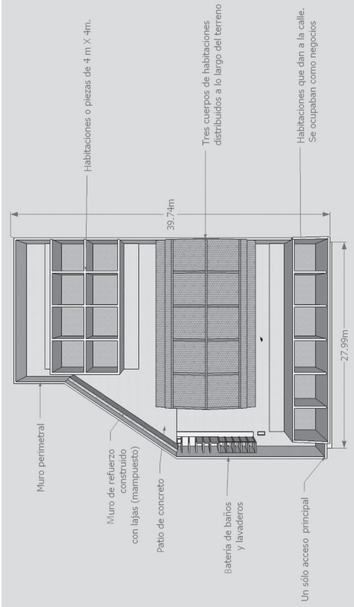
Vista de planta mesón San Rafael. Diseño arquitectónico: Arq. Óscar Batres Posada, con la colaboración de Leonardo Regalado.
